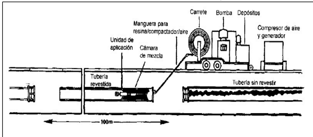
Gráfico 10: Revestimiento con resina epoxi
