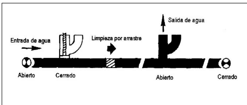
Gráfico 4: Arrastre por esponja
