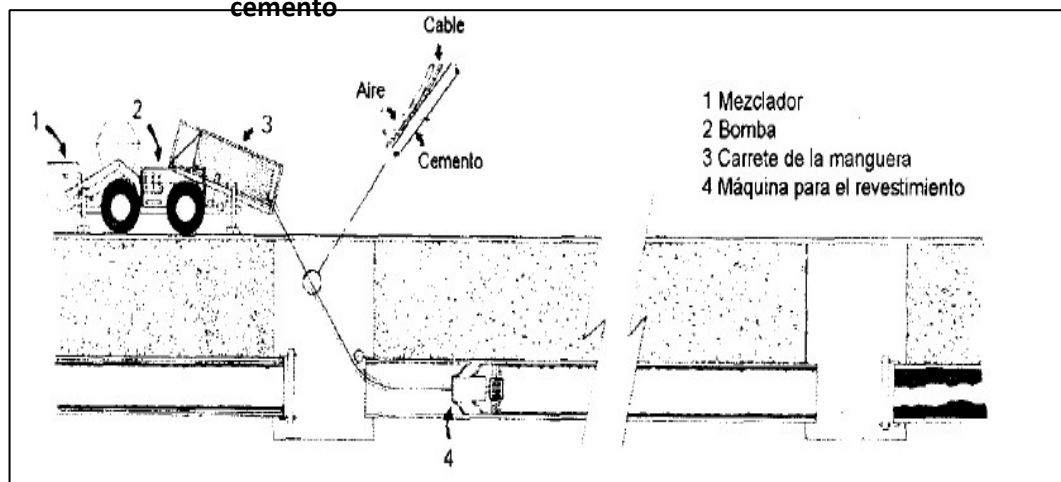
Gráfico 9: Revestimiento con mortero cemento
